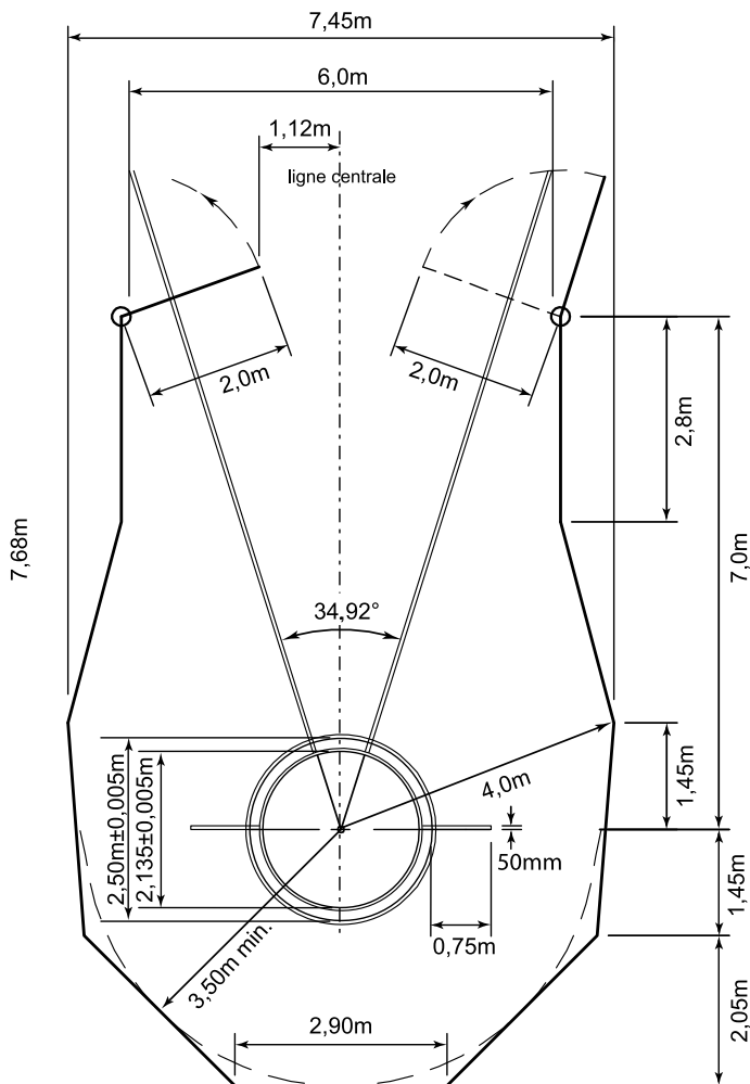
[Schéma 22 - Cage pour le Lancer du Marteau et du Disque avec cercles concentriques (en configuration Marteau)]
