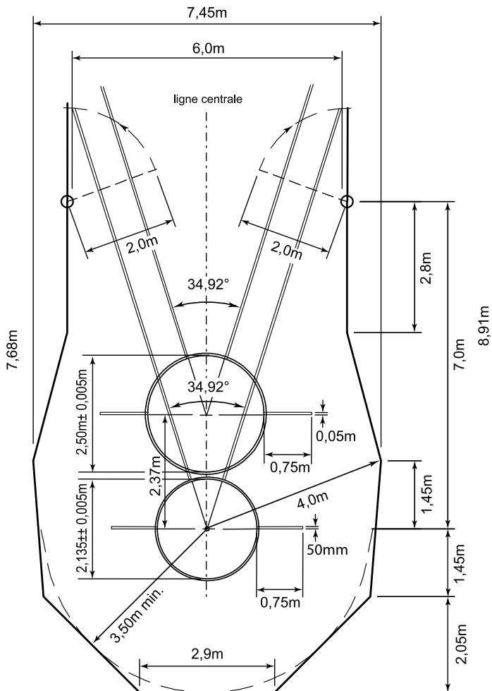
[Schéma 24 - Cage pour le Lancer du Marteau et du Disque avec cercles séparés]
