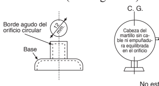
Figura 21.- Aparato que se sugiere para comprobar el centro de gravedad de la cabeza del martillo
